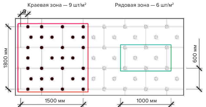
Рис. 33. Рекомендуемая схема расположения тарельчатых дюбелей на плоскости фасада в зависимости от высоты здания
