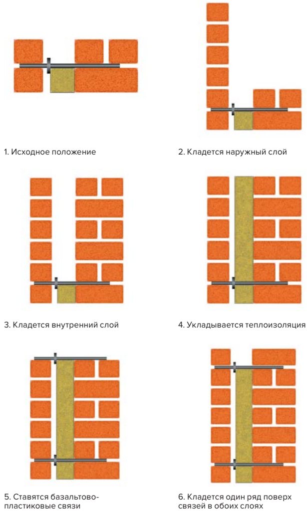
Рис. 8. Последовательность монтажа
