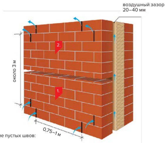
Рис. 17. Обеспечение притока и оттока воздуха при помощи продухов в конструкции слоистой кладки
