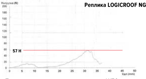
Прочность сварного шва на разрыв, Н/50мм
