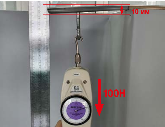
Рейка ТЕХНОНИКОЛЬ
